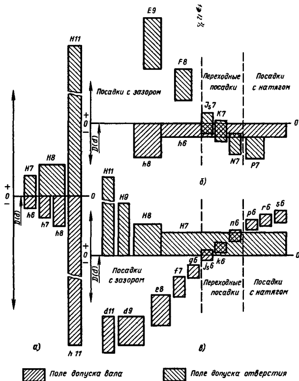
Рис. 15. Посадки предпочтительного применения: а — образованные соединением основных валов и основных отверстий, б — в системе вала; в — в системе отверстия
