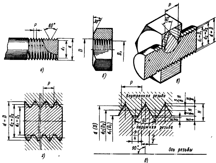
Рис. 1. Наружная (а), внутренняя (б) резьба, соединение болта с гайкой (в) и параметры резьбы (г и д)
