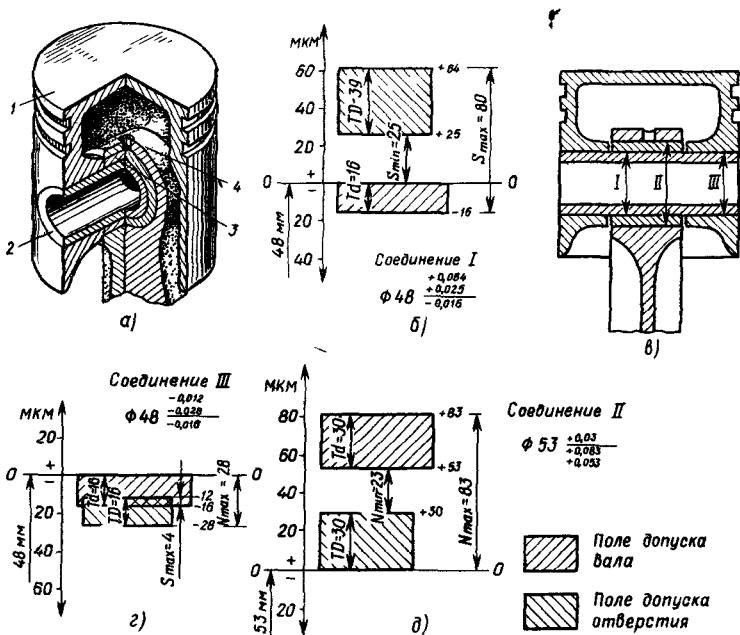
Рис. 5. Детали поршневой группы в сборе (а) и их сборочный чертеж (в), обозначения на чертеже соединения деталей и схема расположения полей допусков для посадки с зазором (б), переходной посадки (г) и посадки с натягом (д): 1 – поршень, 2 – поршневой палец, 3 – втулка верхней головки шатуна, 4 – шатун
