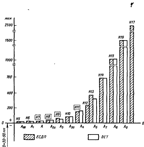
Рис. 3. Поля допусков основных отверстий
