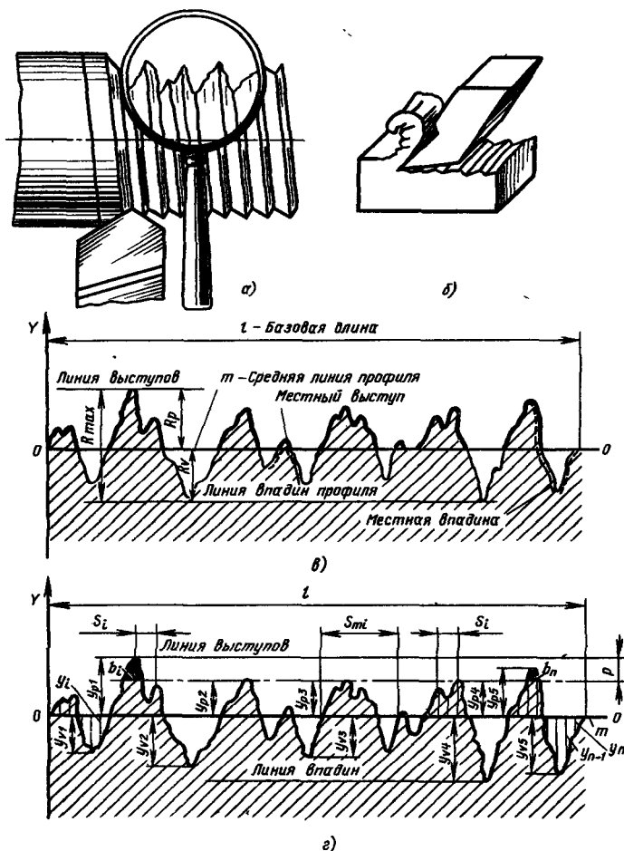
Рис. 4. Шероховатость поверхности при токарной обработке (а), при строгании (б) и профилограммы обработанной поверхности (в и з)
