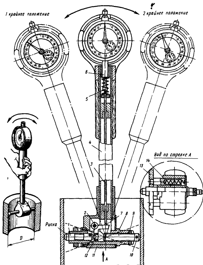
Рис. 6. Индикаторный нутромер
