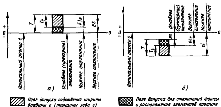
Рис. 7. Расположение полей допусков ширины впадины e втулки (а) и толщины зуба s вала (б)
