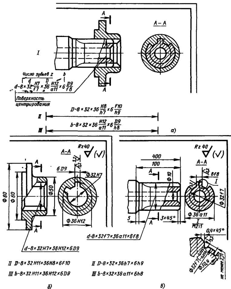
Рис. 5. Обозначение допусков и посадок прямого шлицевого соединения на сборочном чертеже (а) и на рабочих чертежах деталей (б и в); варианты обозначения при центрировании:
