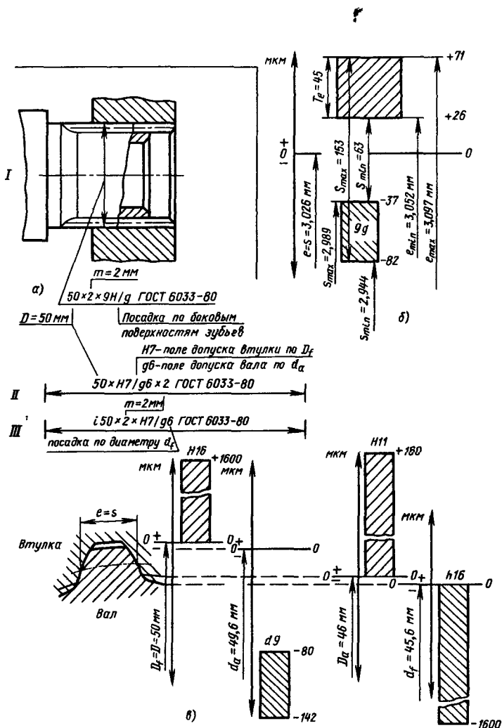
Рис. 9. Обозначение допусков и посадок эвольвентного шлицевого соединения при центрировании:
