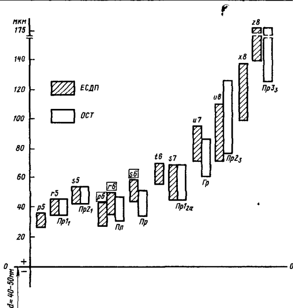
Рис. 7. Поля допусков валов посадок с натягом
