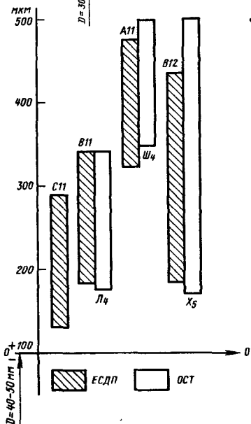
Рис. 10. Поля допусков отверстий посадок с зазором
