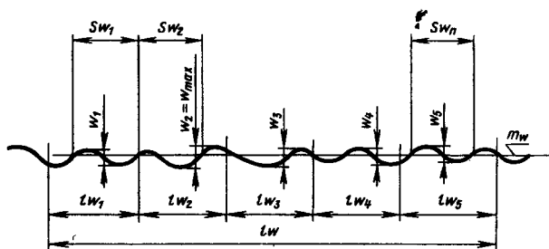
Рис. 6. Параметры волнистости поверхности:
