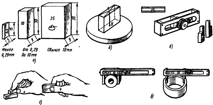
Рис. 2. Плоскопараллельные концевые меры длины:
