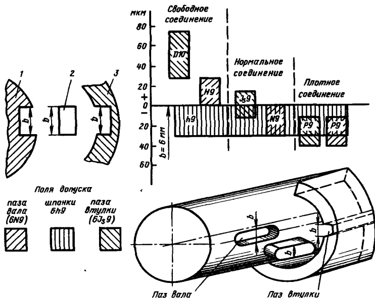
Рис. 2. Схема расположения полей допусков шпоночного соединения с призматической шпонкой:
